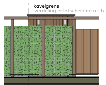
Aanzicht parkeerstraat
