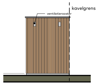
Voorgevel berging
