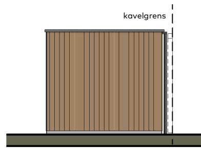
Rechterzijgevel berging
