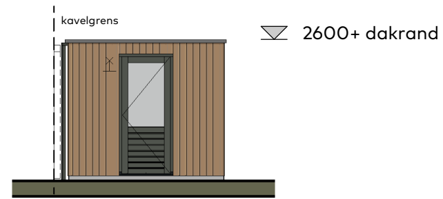
Linkerzijgevel berging
