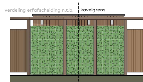
Aanzicht parkeerstraat
