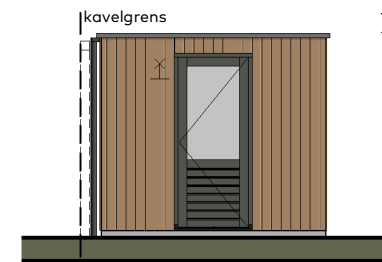
Linkerzijgevel berging
