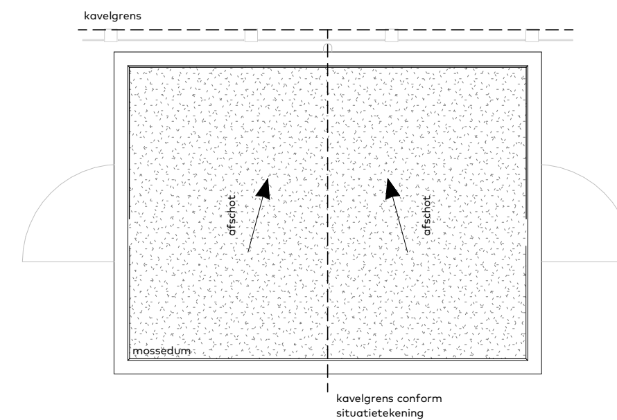
Dak aanzicht
