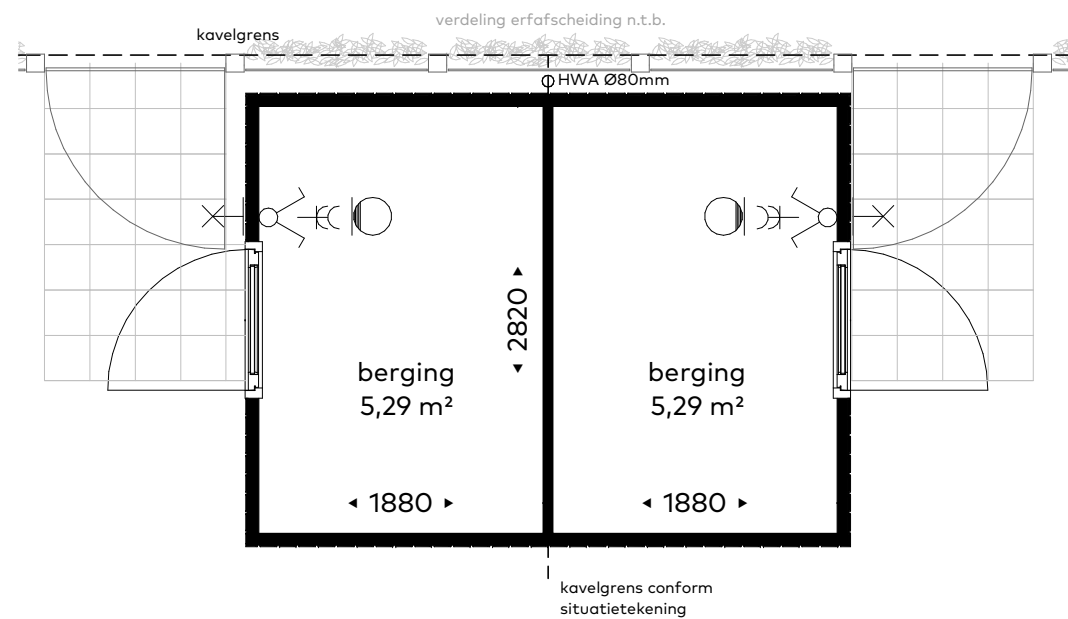
Begane grond
