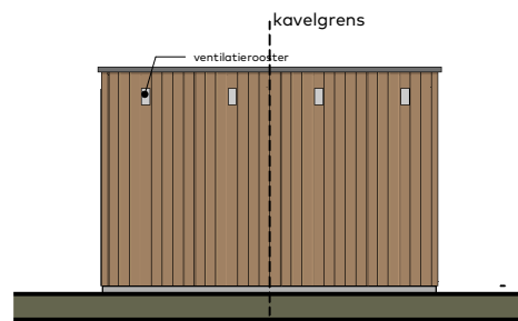
Vorgevel berging
